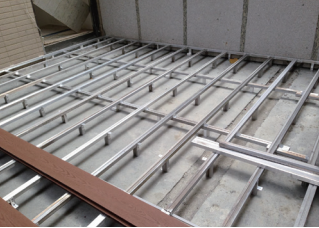
外部用スチール製根太と専用取付金具を使用した施工例
