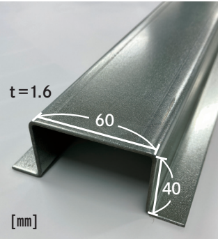
外部用スチール製根太
